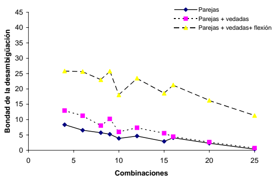
Figura 3: Estudio sobre ternas teóricas: c) con ambigüedad sólo por la izquierda
