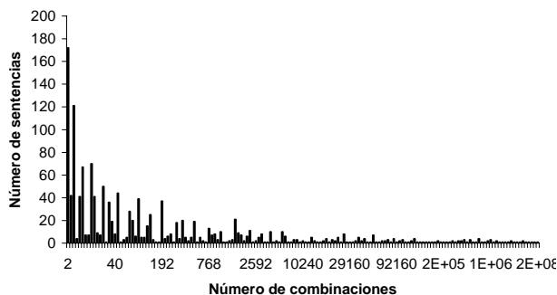
Figura 5: Distribución del número de combinaciones por sentencia en el texto
