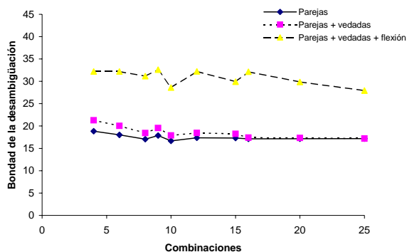
Figura 2: Estudio sobre ternas teóricas: b) con ambigüedad sólo por la derecha
