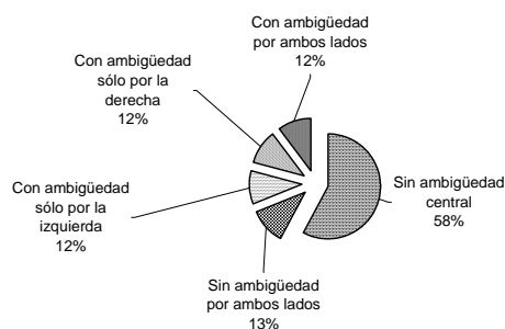
Figura 6: Distribución de los tipos de ternas en el texto
