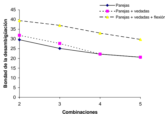
Figura 4: Estudio sobre ternas teóricas: d) sin ambigüedad por ambos lados
