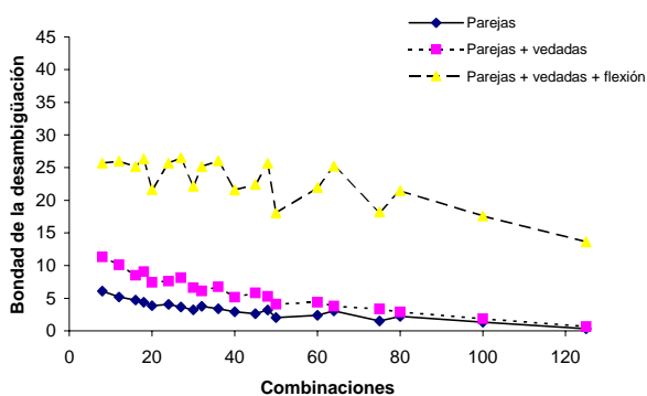
Figura 1: Estudio sobre ternas teóricas: a) con ambigüedad por ambos lados
