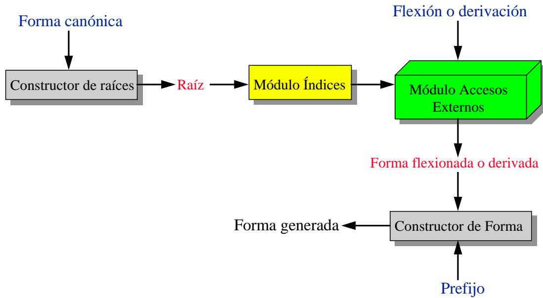
Figura 6: Esquema del generador
