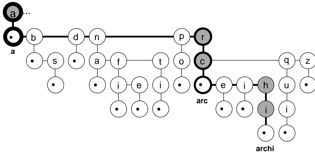
Figura 5: Árbol de prefijos
