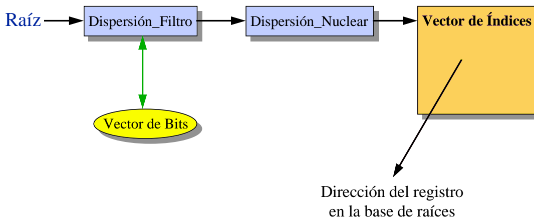
Figura 1: Módulo de índices
