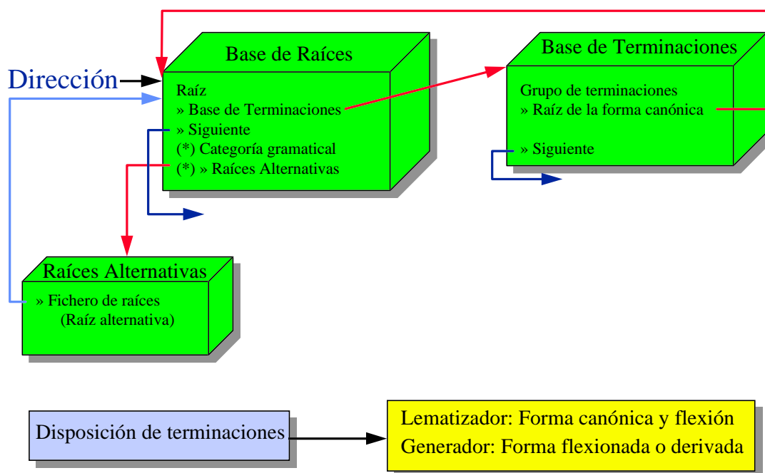
Figura 2: Módulo de accesos externos
