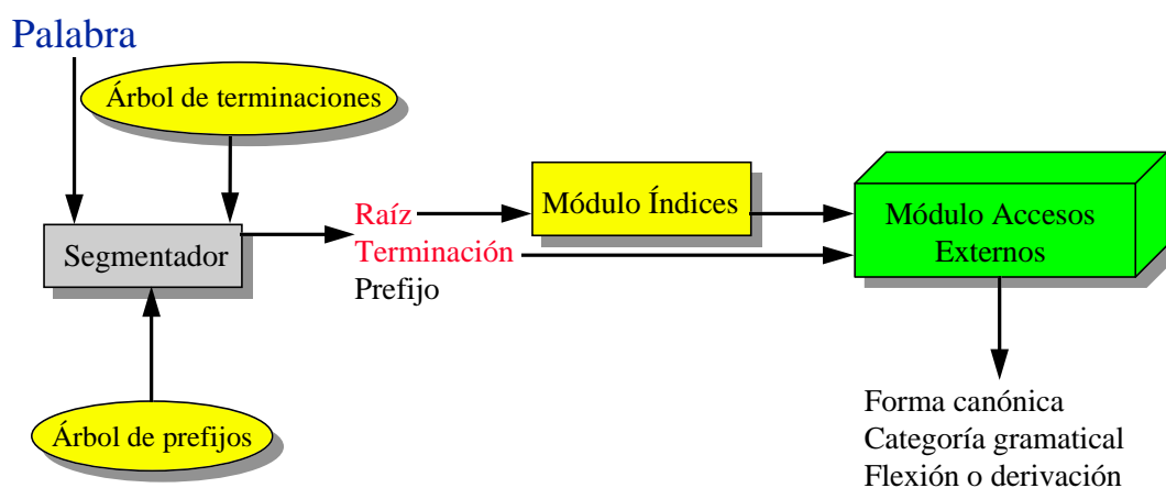
Figura 3: Esquema del lematizador
